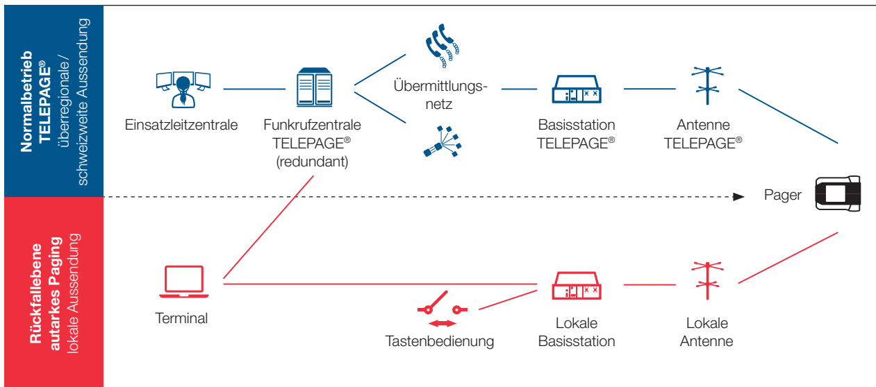
TELEPAGE®-Funkrufnetz mit Rückfallebene Autarkes Paging
